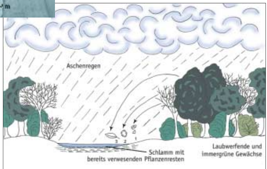
Rekonstruktion einer überfluteten Aulandschaft. Mit dem Aschenregen gelangen Knospen, Knospenschuppen (1), Blütenteile (2) und Blätter immergrüner Gehölze (3) in den Schlamm, der bereits verwesende Pflanzenreste enthält.
